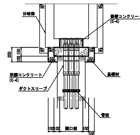
平面図 (A-A)
