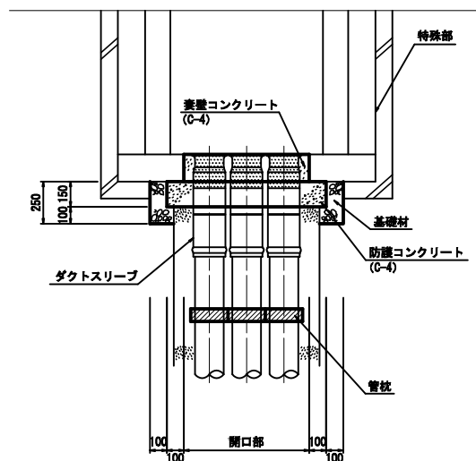
平面図 (A-A)
