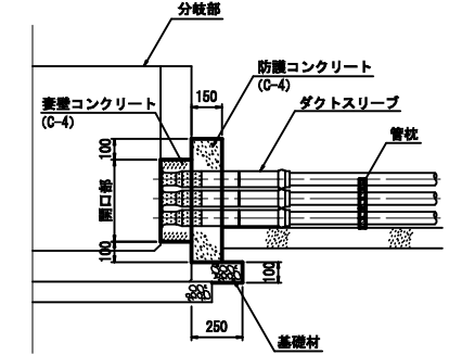
断面図 (B-B)
