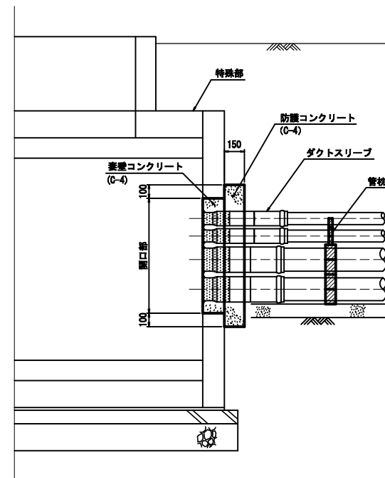
断面図 (B-B)
