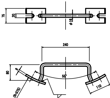
梯子フック詳細図 SS400 HDZT77
