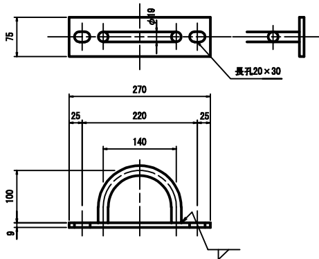
プーリングフック詳細図 SS400 HDZT77
