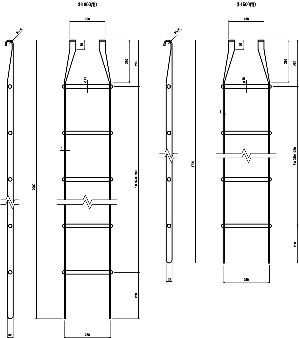
梯子詳細図 SS400 HDZT77
