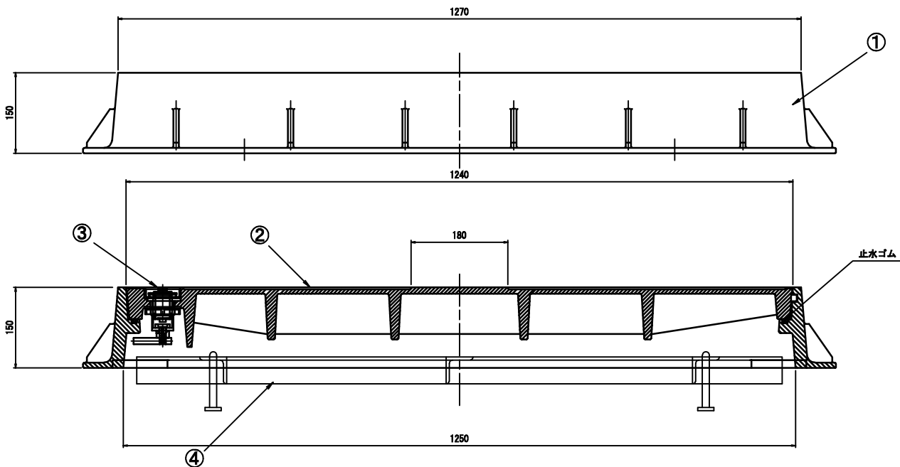
A-A 断面
