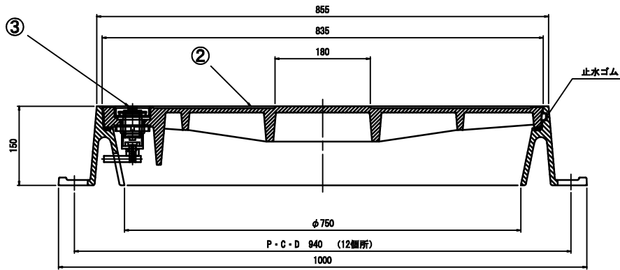
A-A 断面
