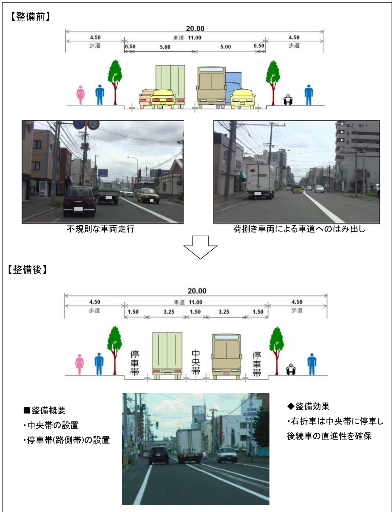
図 4-7 中央帯・停車帯実施事例
