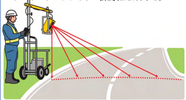
レーザープロファイラー計測(LP2100など)
