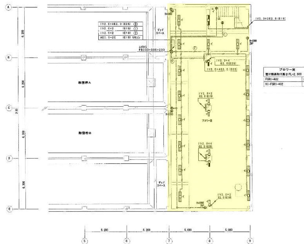
地下2階平面図
