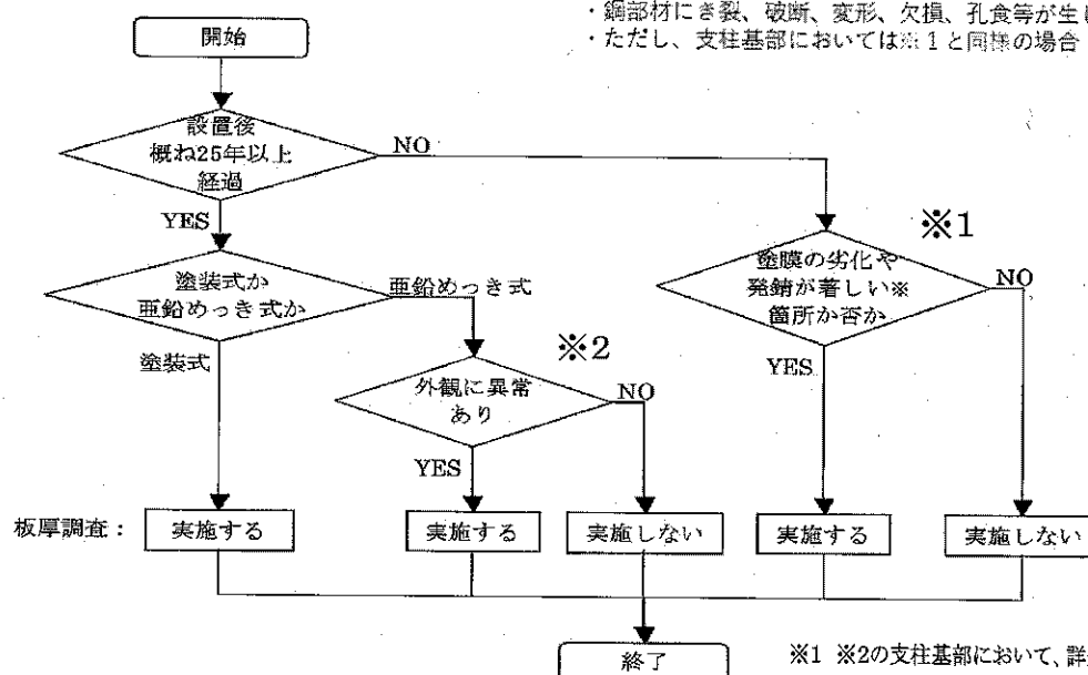
図-解 8-13 板厚調査を実施する附属物の選定フロー
