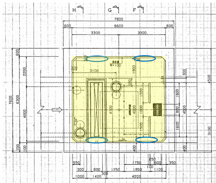
堰室平面図
