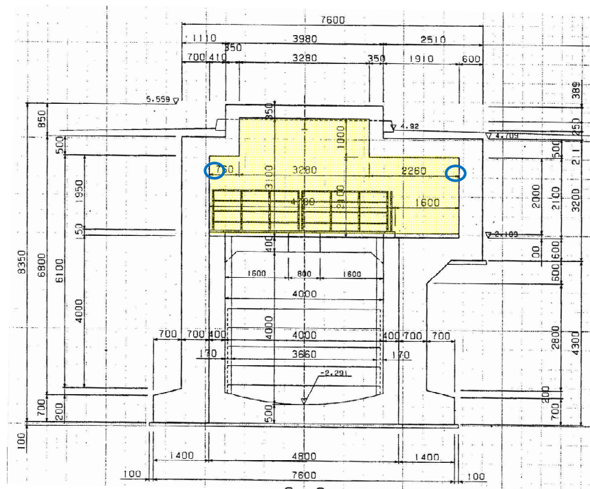
堰室立面図
