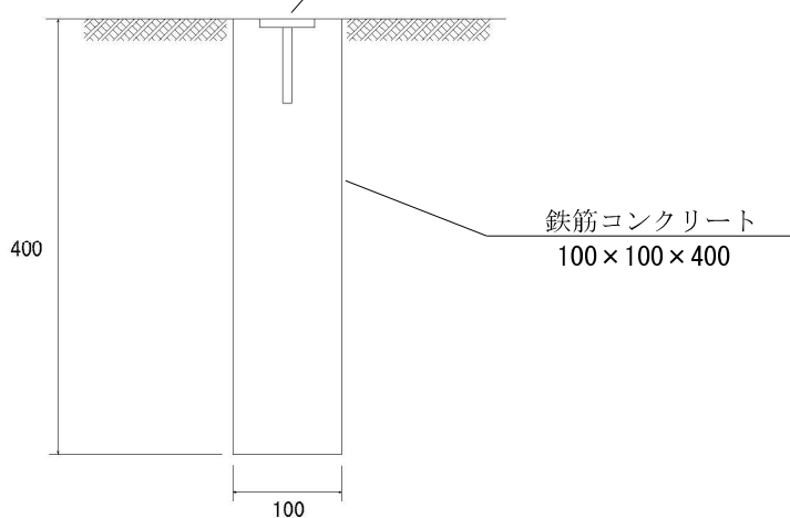
【側面図】
