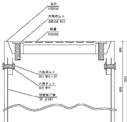
【公共基準点用鉄蓋（金母・塩ビ管共）断面図】
