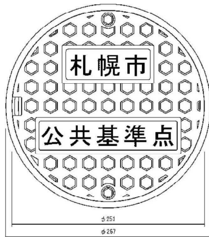
【平面図】
