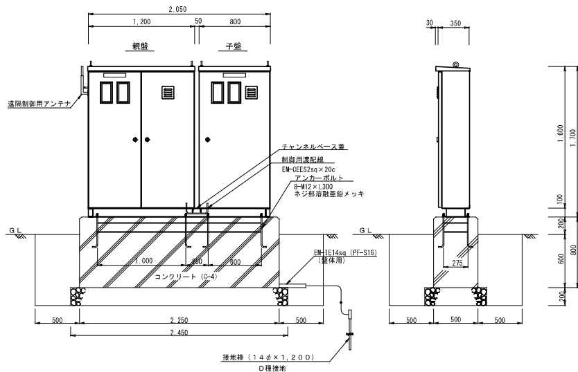
外形圖 基礎圖 S=1:20
