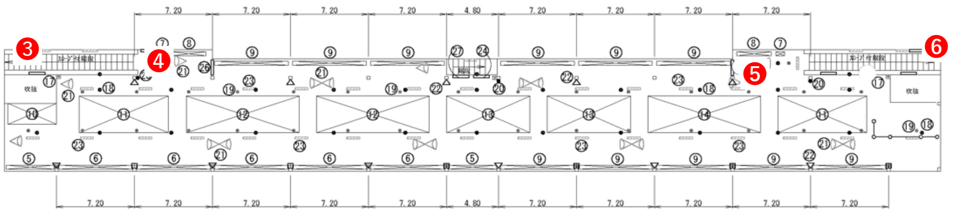
地階平面図
