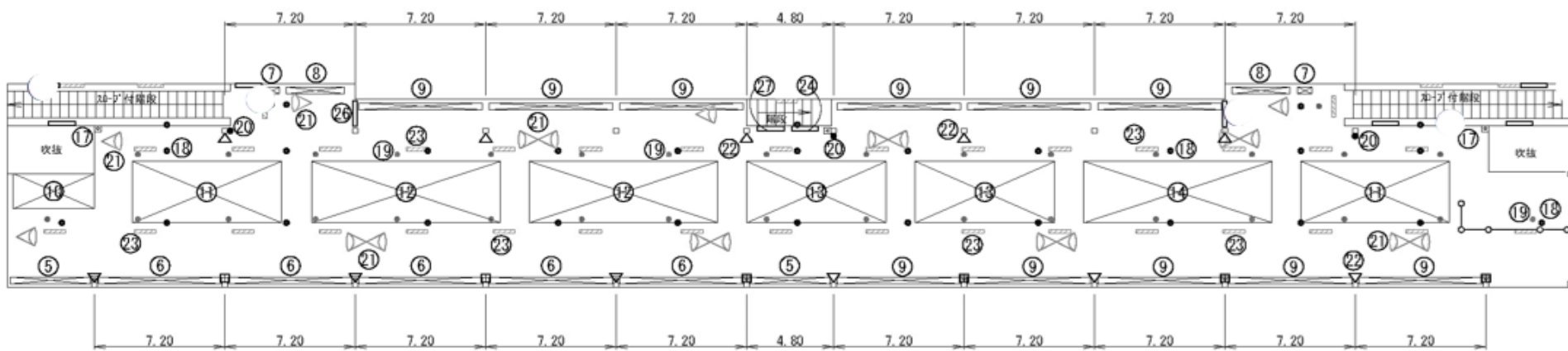
地階平面図
