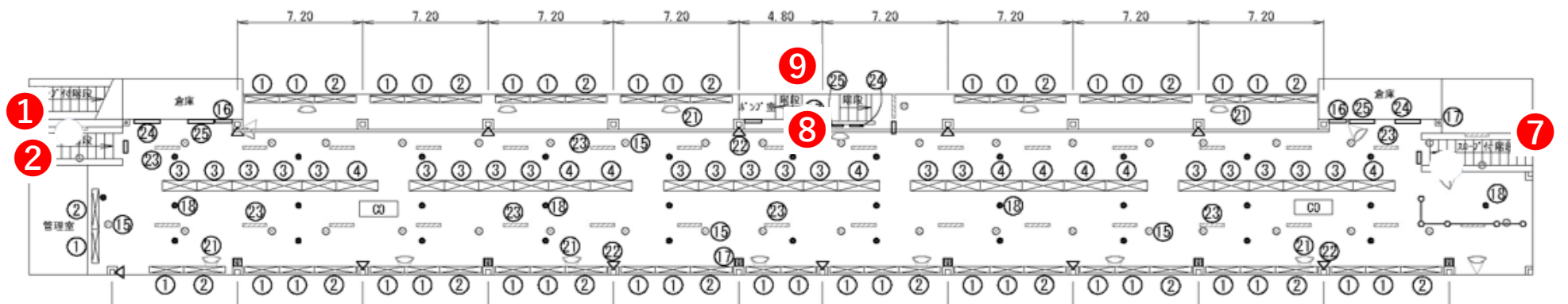
地階平面図
