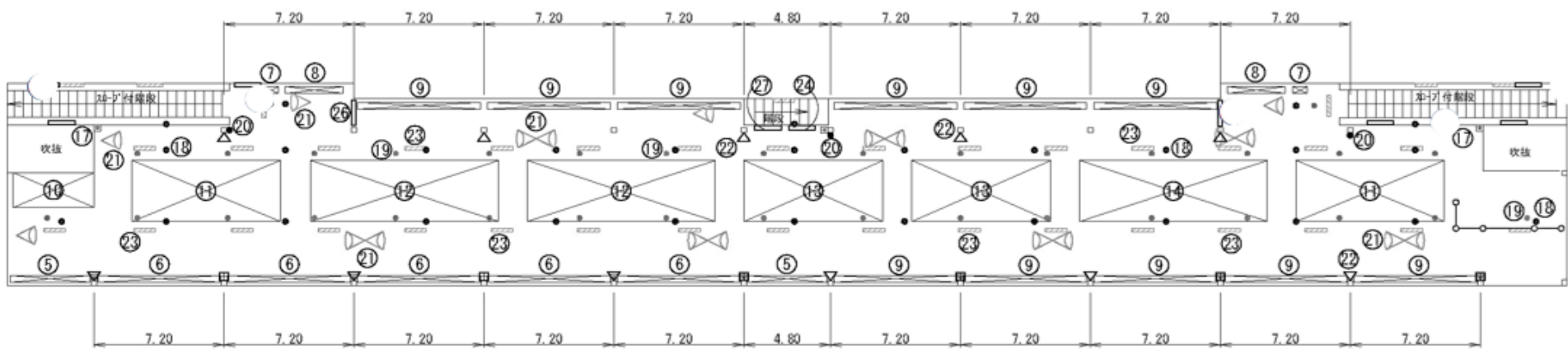
地階平面図
