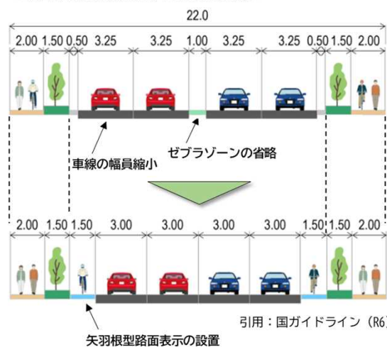
図 道路空間の再分配による整備イメージ
