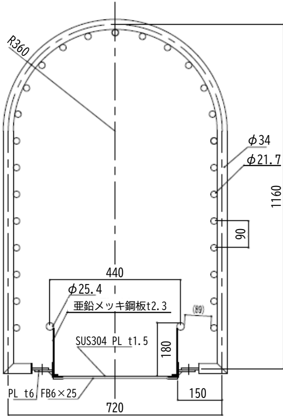
滑面断面図
