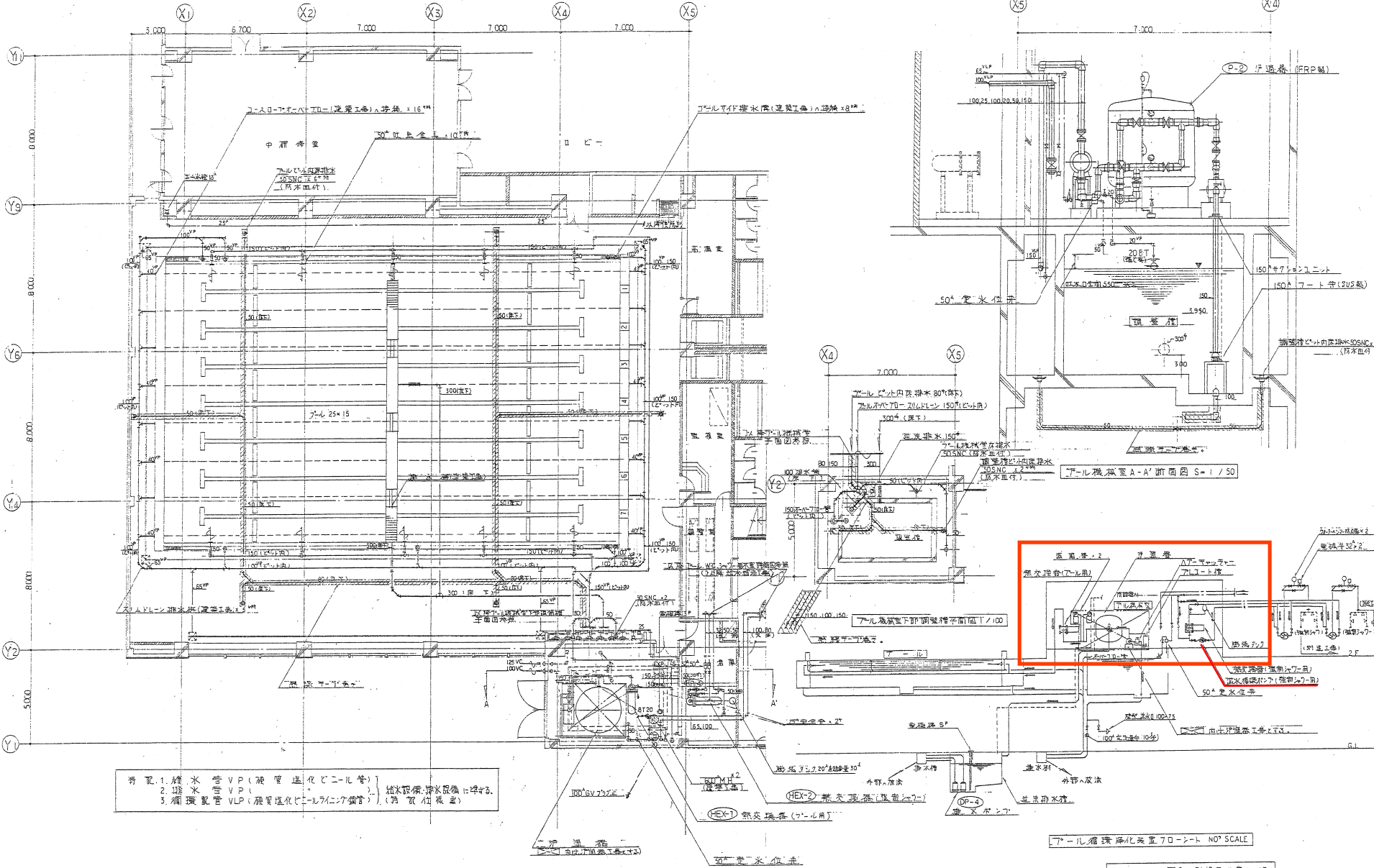
7°-11-1 脱臭室平面図 S=1/50
