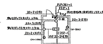
電気配線図 S=1:100
