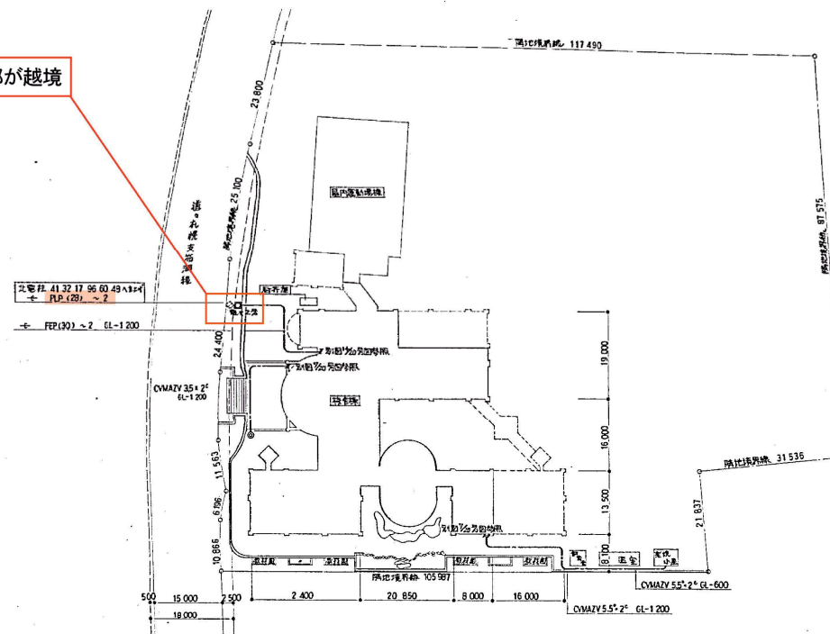
配置図 S=1:500
