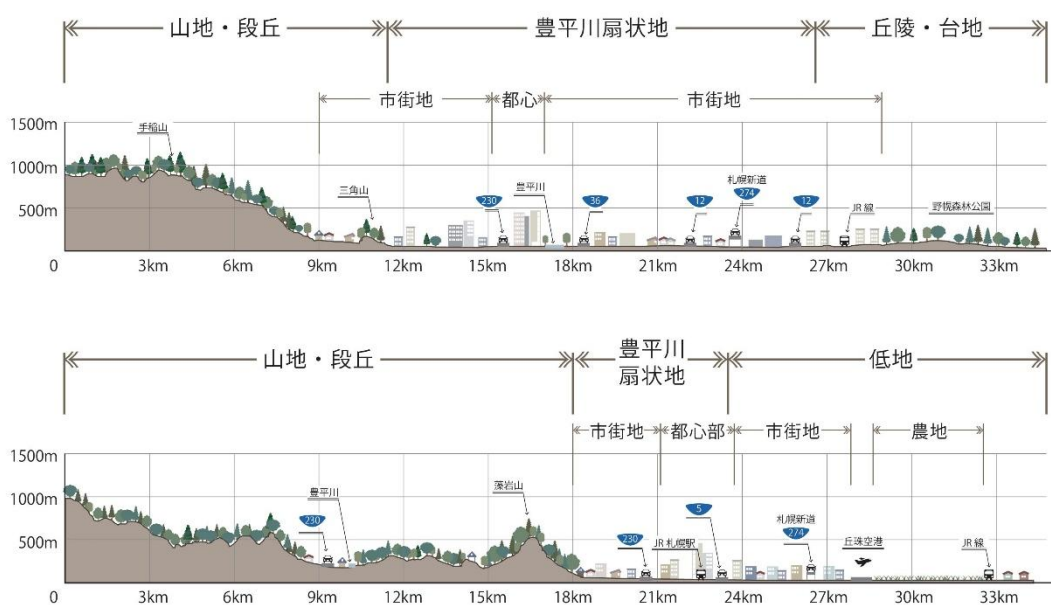
図 地形断面図
