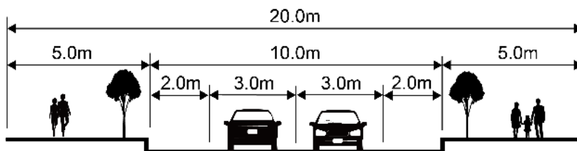
図1 幅員構成
