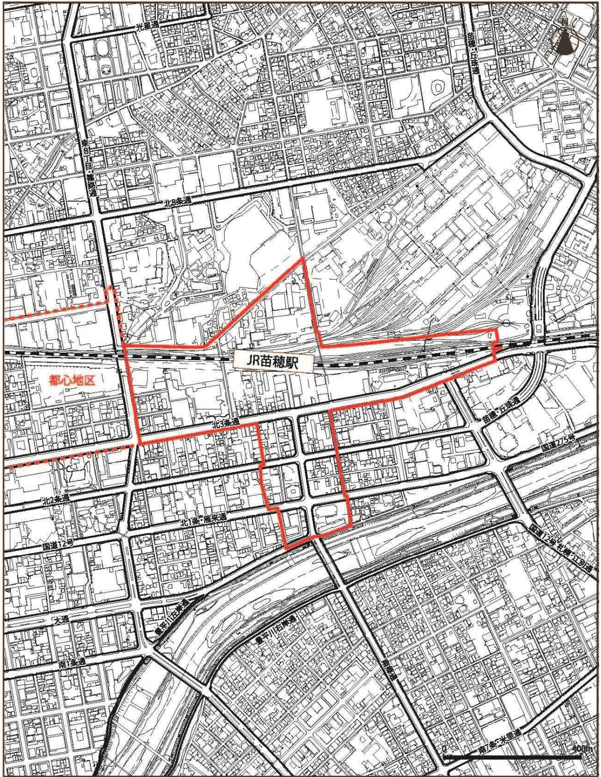
札幌市都市再開発方針 苗穂駅周辺地区 2号地区
