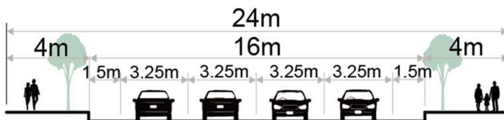
図1 幅員構成
