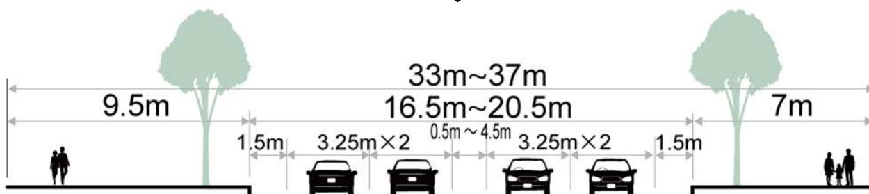
図2 幅員構成
