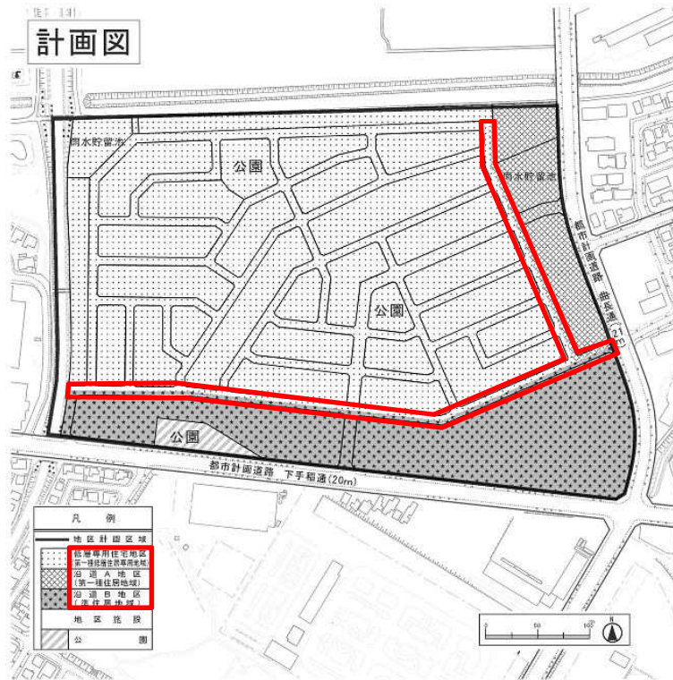
計画図
