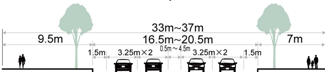
図2 幅員構成
