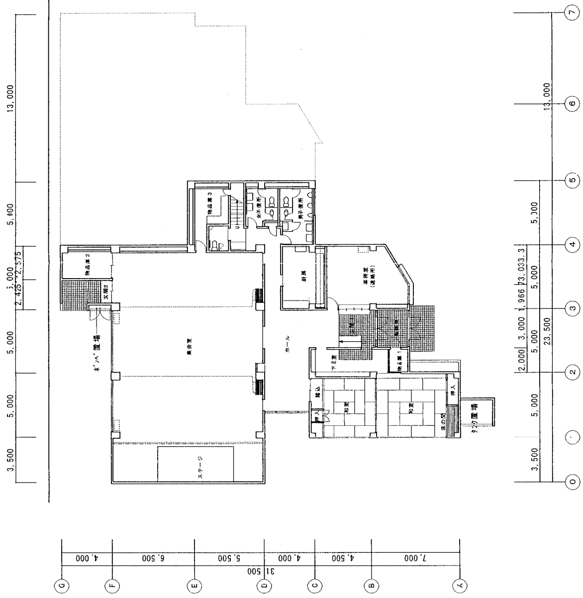
1階平面図 1:200
