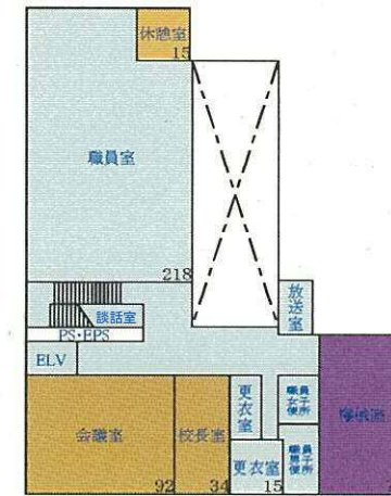
2 階 平面 図
