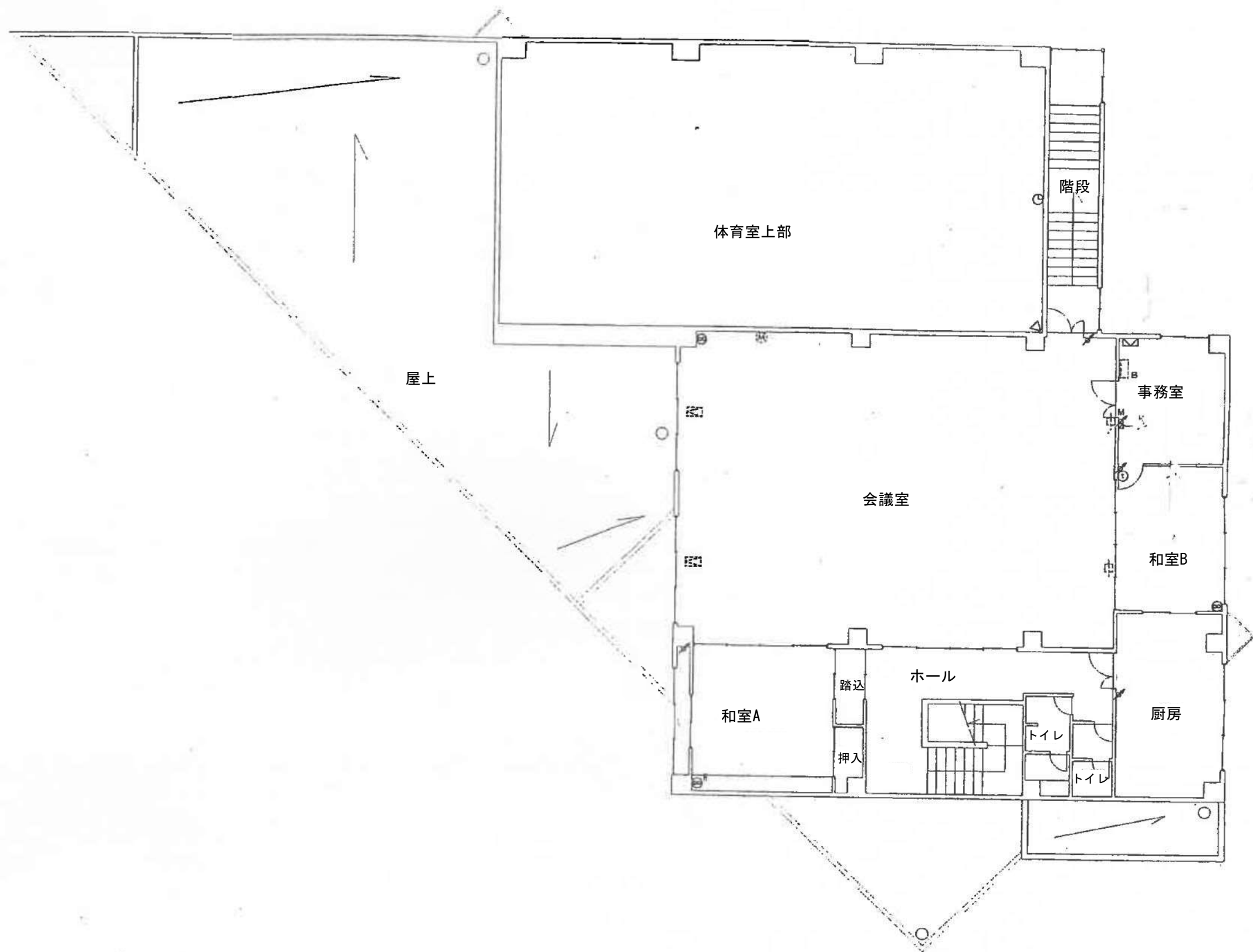
2階平面図
