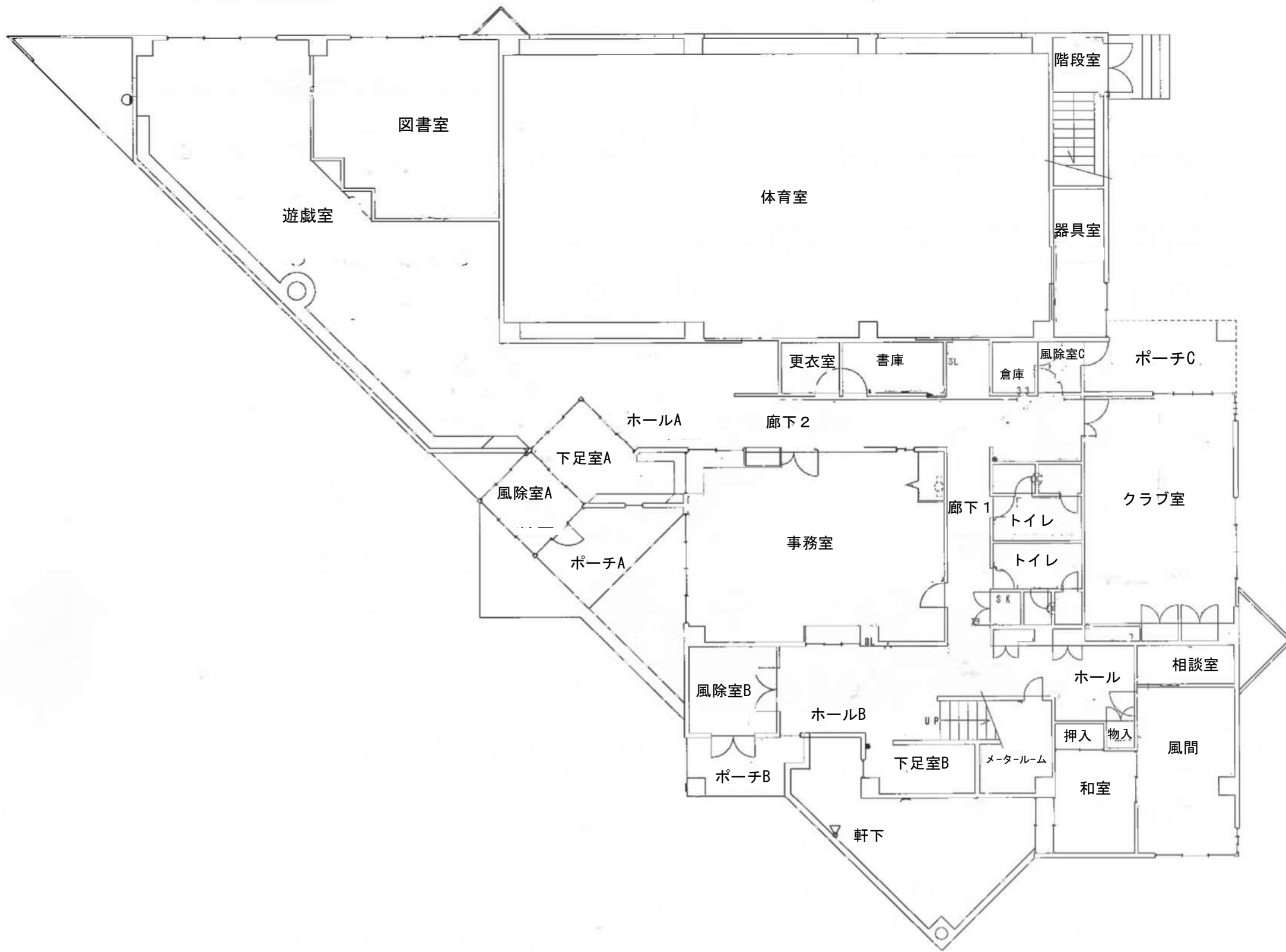
1階平面図
