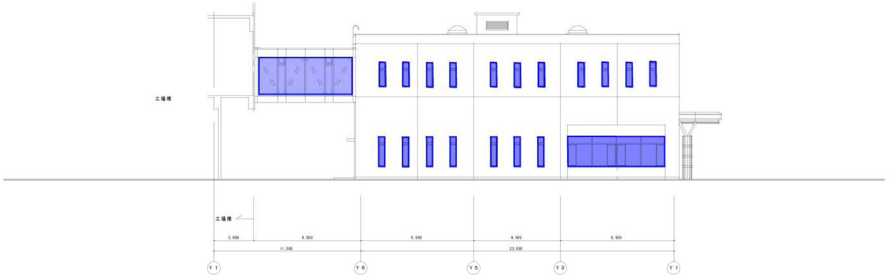
左側面図 1/200
