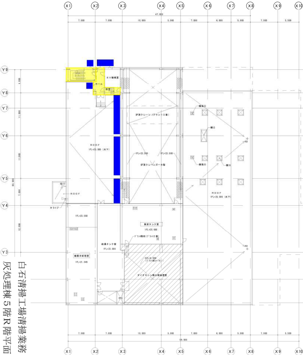
5階平面図 1/250
