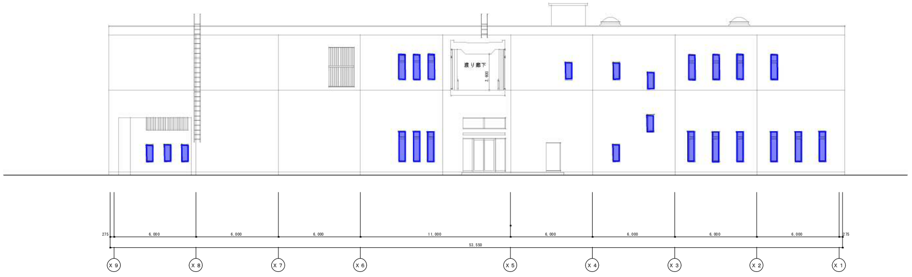
背面図 1/200
