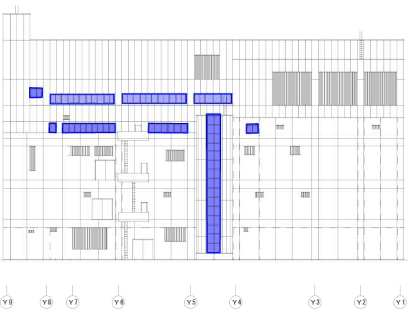
南立面图
