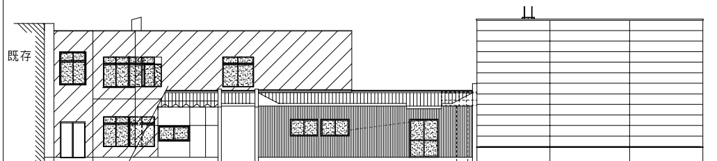
北側立面図
