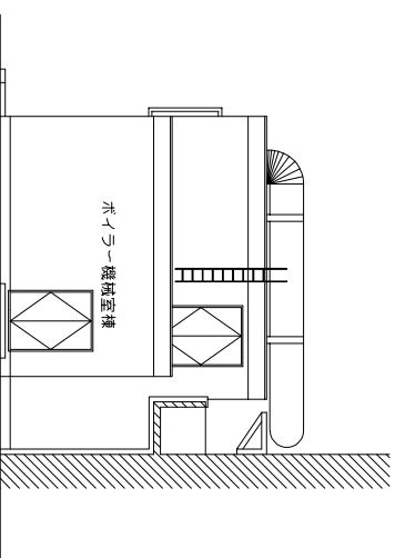
南立面図
