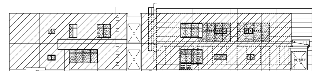
東側立面図
