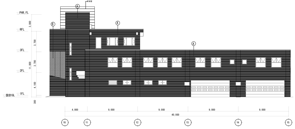
北立面図
