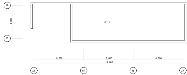
屋根伏図
