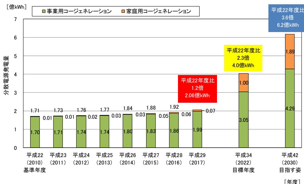
図 3-5 分散電源発電量の推移
