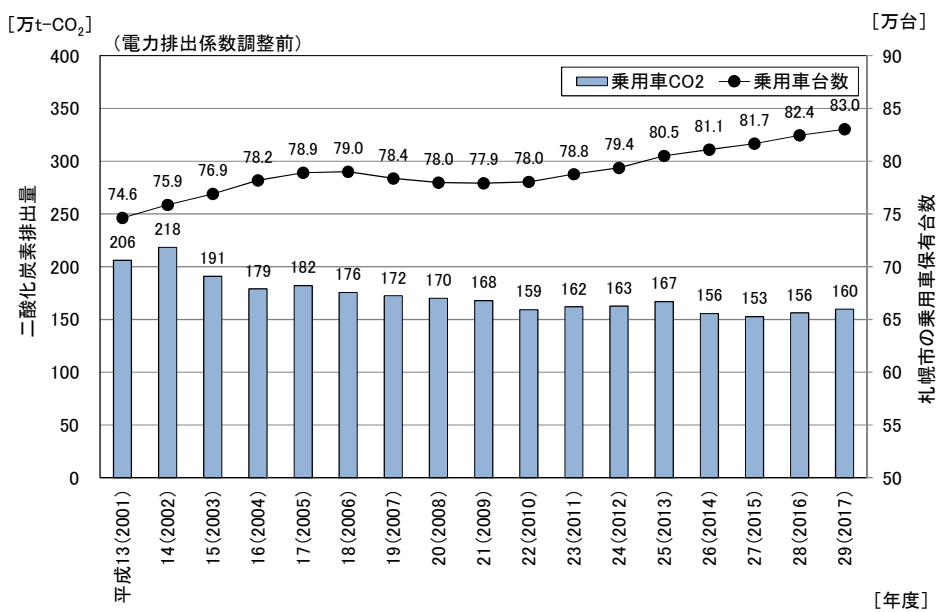
図 6-3-7 乗用車の二酸化炭素排出量と台数の推移
