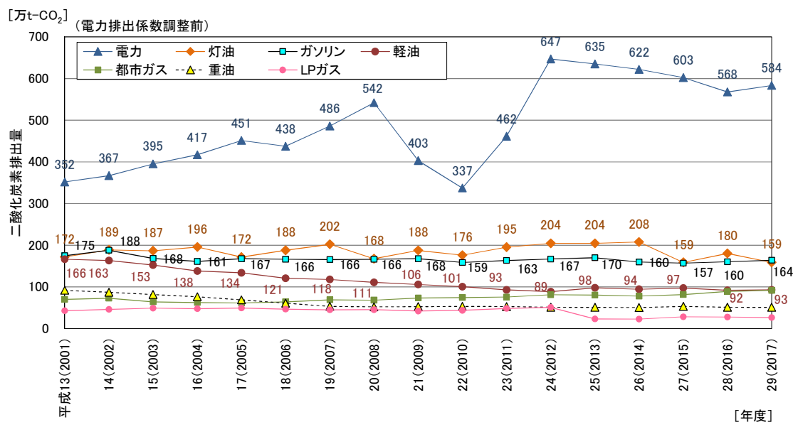
図 4-4-2 二酸化炭素排出量のエネルギー種別推移(その2)
