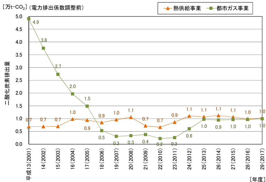
図 6-6-7 エネルギー転換部門の二酸化炭素排出量の推移(事業別)
