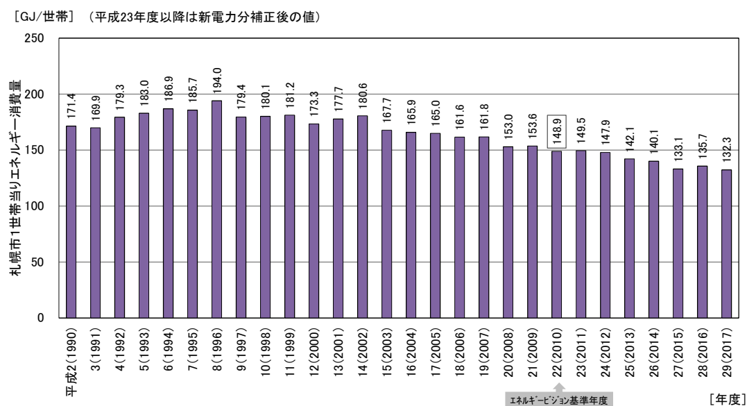
図 2-1-3 札幌市内の1世帯当たりのエネルギー消費量の推移
