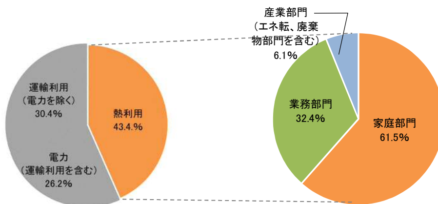
図 2-3-3 熱利用エネルギー消費量の部門別内訳 (平成 29 年度速報値)
