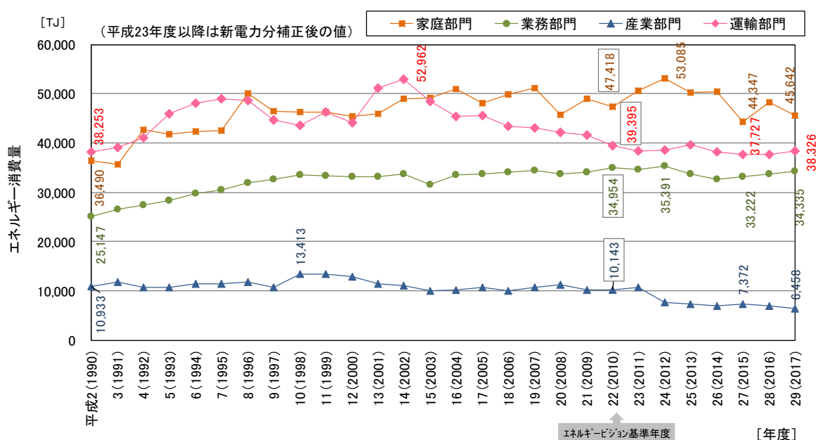
図 2-1-4 エネルギー消費量の推移(部門別)
