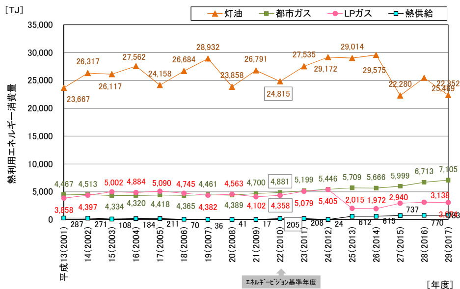
図 6-1-4 家庭部門の熱利用エネルギー消費量の推移(エネルギー種別)
