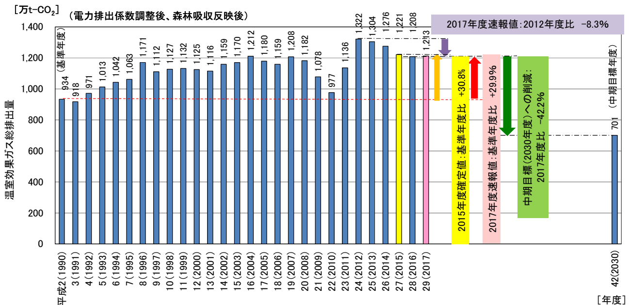
図4-1-1 温室効果ガス総排出量の推移
