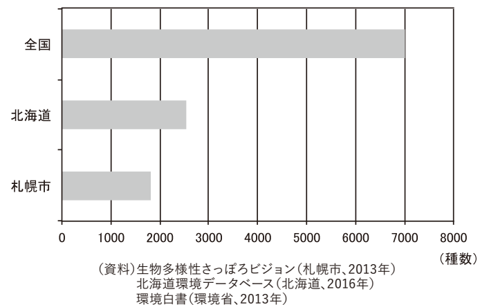
図2-4-4 札幌市・北海道・全国の植物
