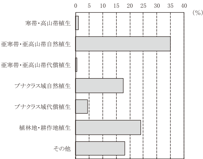
図2-4-2 札幌市周辺の現存植生
