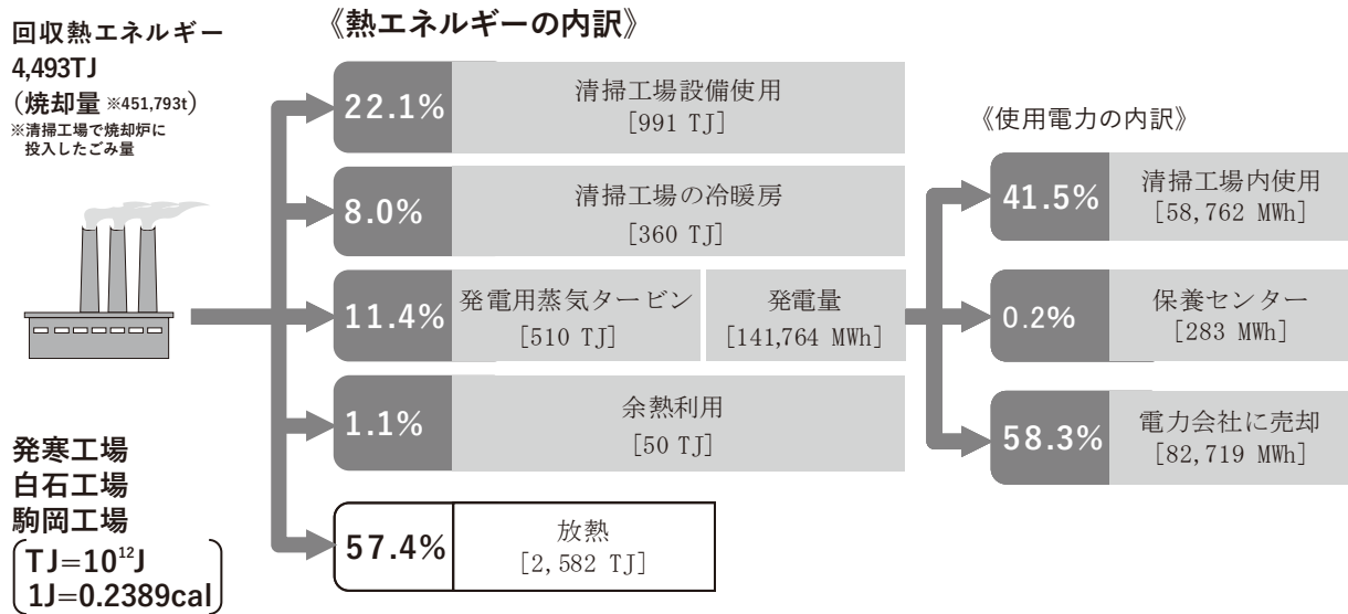
図2-3-15 清掃工場の熱利用(2019年度実績)
