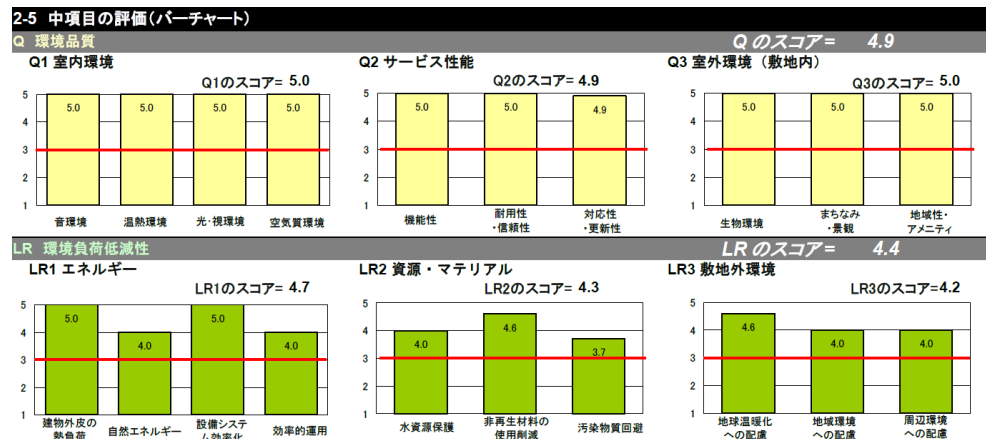
図 4.13.1 「評価結果表示シート」 2-5 の拡大(バーチャートによる表示)
