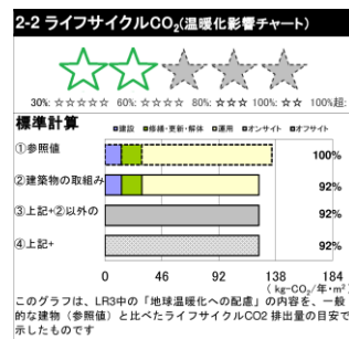
図 4.13.1 2-2 の拡大 (ライフサイクル CO 2 と緑星による表示)
