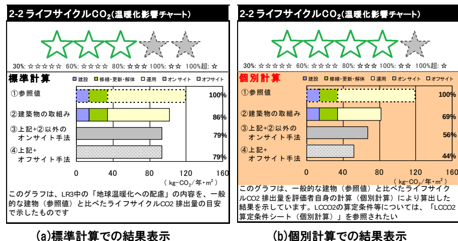
図Ⅲ. 2.3 CASBEE 札幌におけるライフサイクル CO 2 (温暖化影響チャート)の表示
