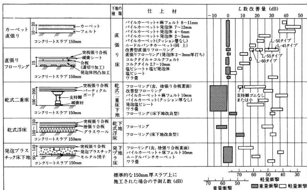
■参考2) 各種仕上げ材のL値改善量
