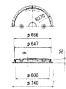
蓋(内蓋)φ600 詳細図 密閉型マンホールカバー (完全防水型、継付)
