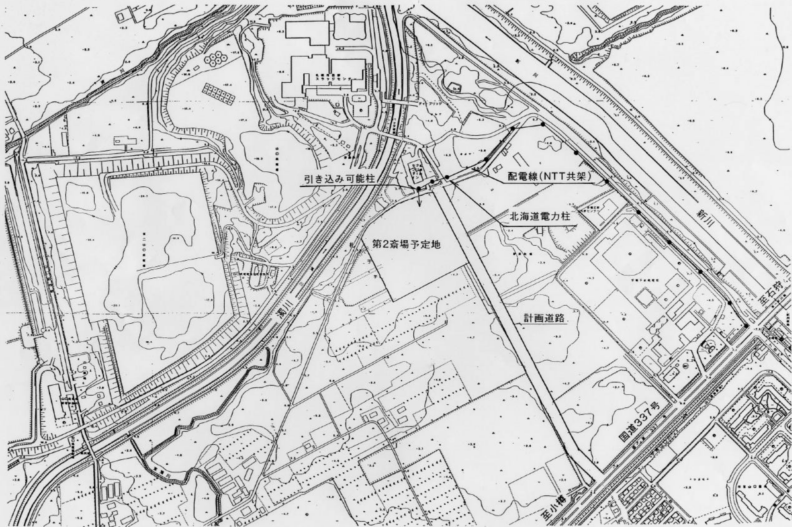
別紙-9 電力・電話引き込み計画図(S=1/5000)
