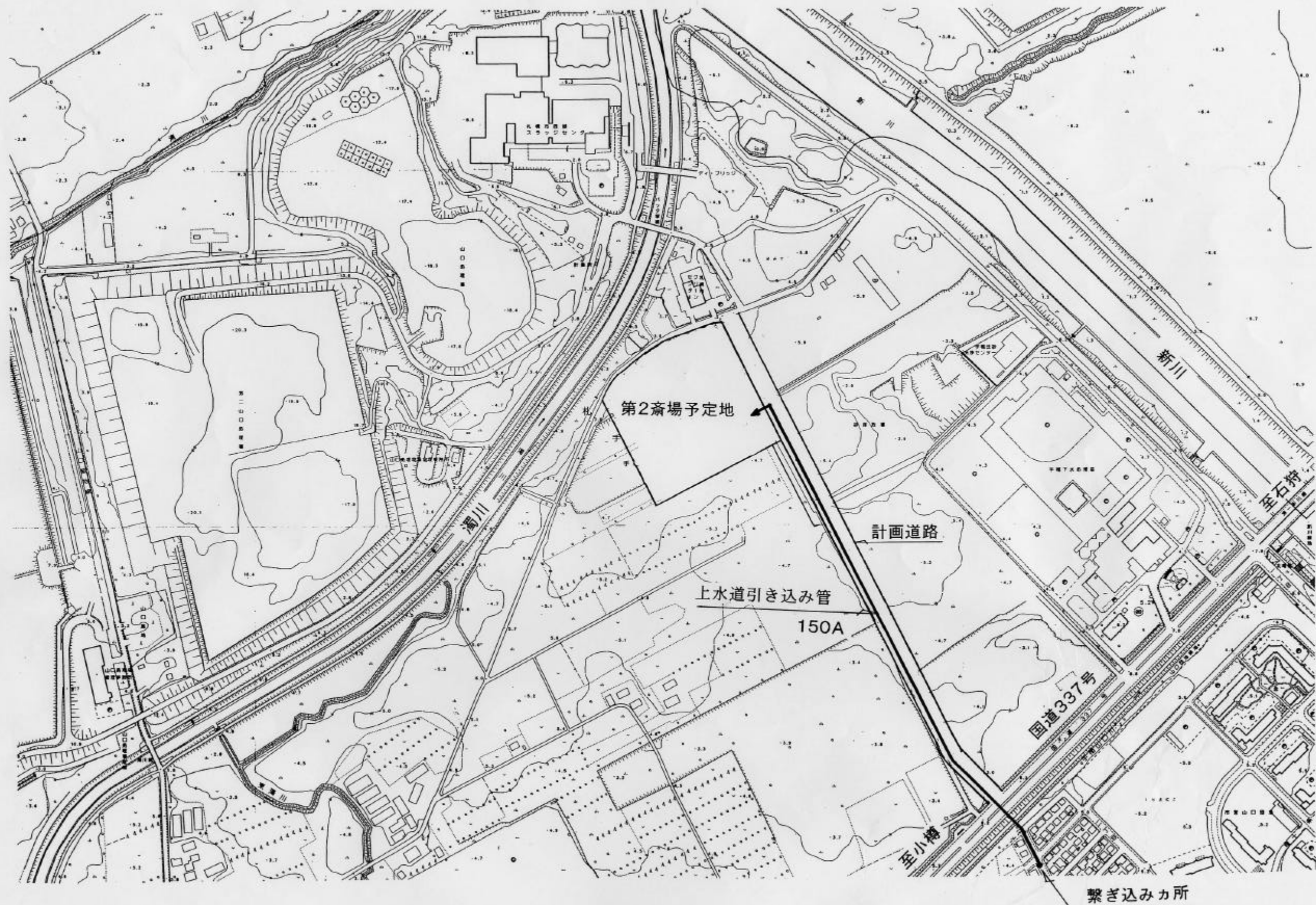
別紙-11 上水道引き込み計画図(S=1/5000)
