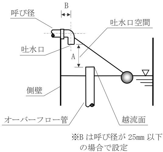
a) オーバーフロー管の管端が上を向いている場合の吐水口空間（断面図）
