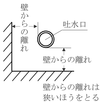
d) 近接壁 2 面の場合の壁からの離れ（平面図）
