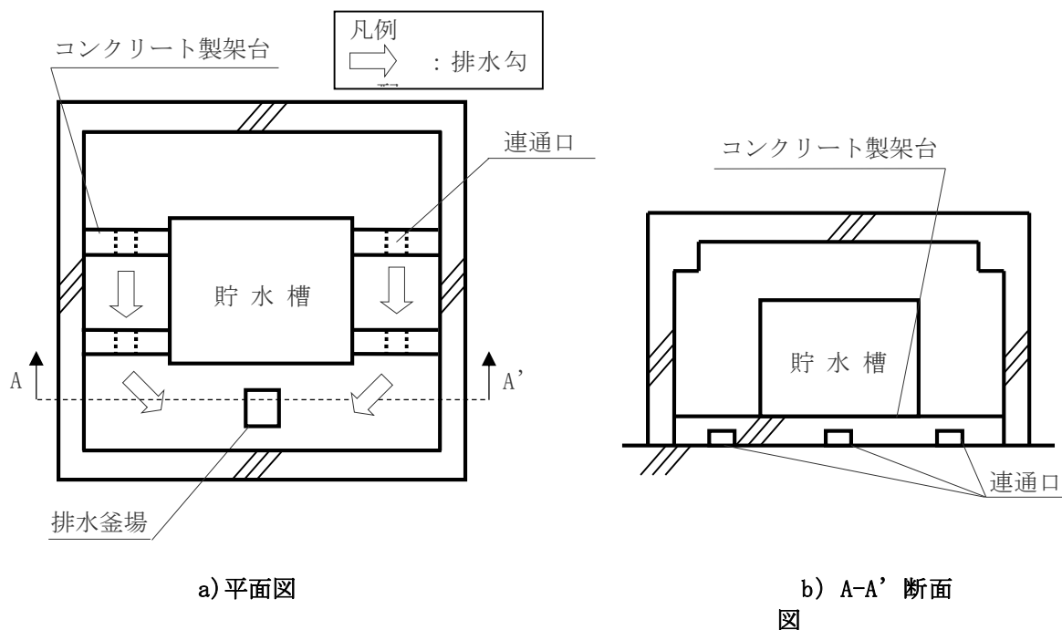
図 2-4 架台の連通口の設置例
