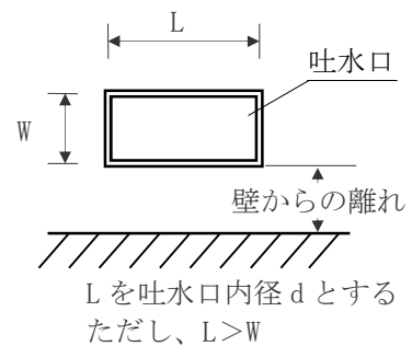
e) 流入口断面が長方形の場合（平面図）
