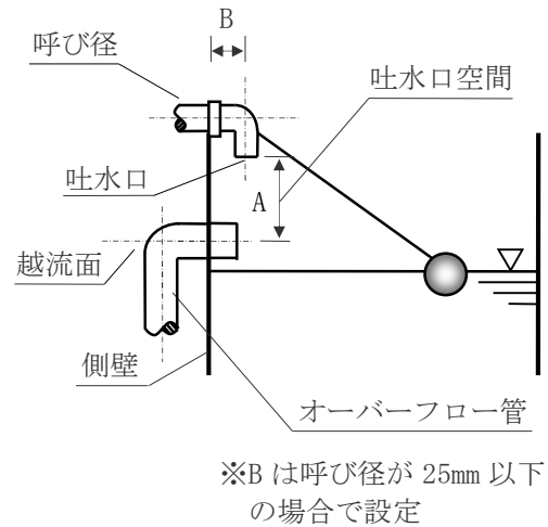
b) オーバーフロー管を水平に取り付けた場合の吐水口空間（断面図）
