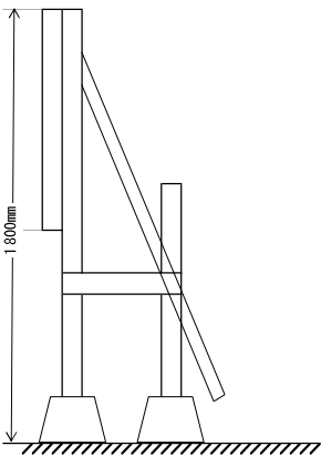
（側面図）
