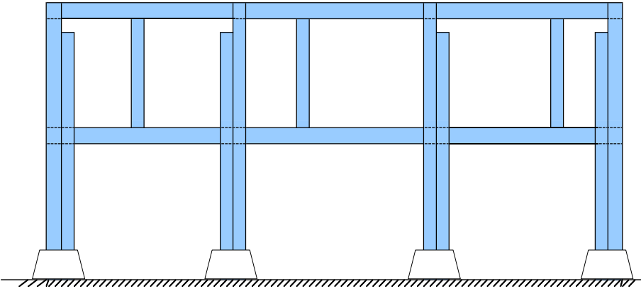
（背面図）
