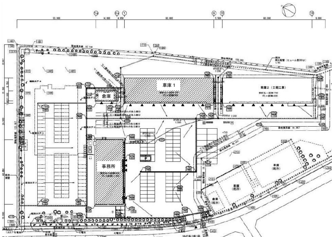
配置図
