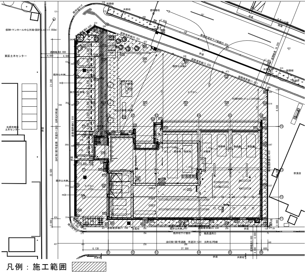
配置図
