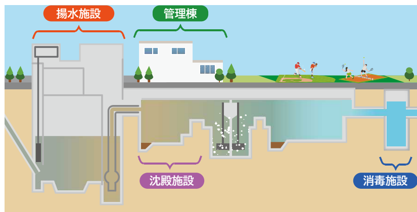
揚水施設(ポンプ施設)
