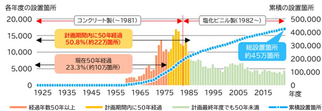
取付管の年度別整備状況
