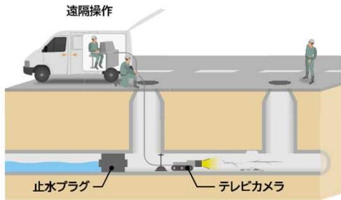
下水道本管のテレビカメラ調査
