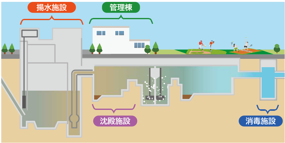
水再生プラザの主な施設
