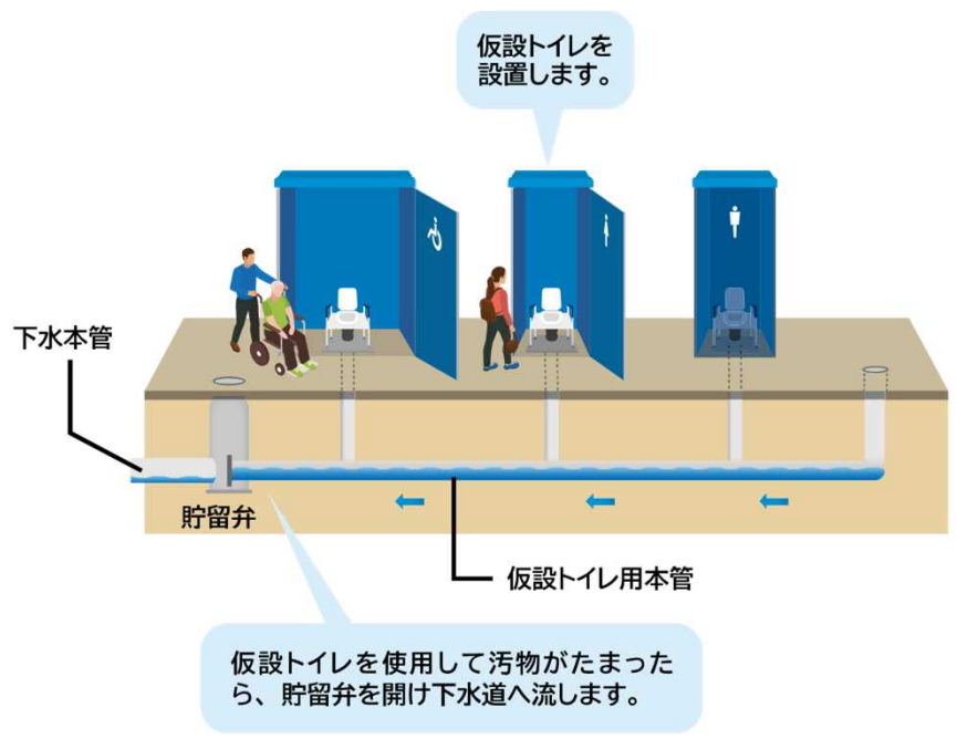
マンホールトイレ
