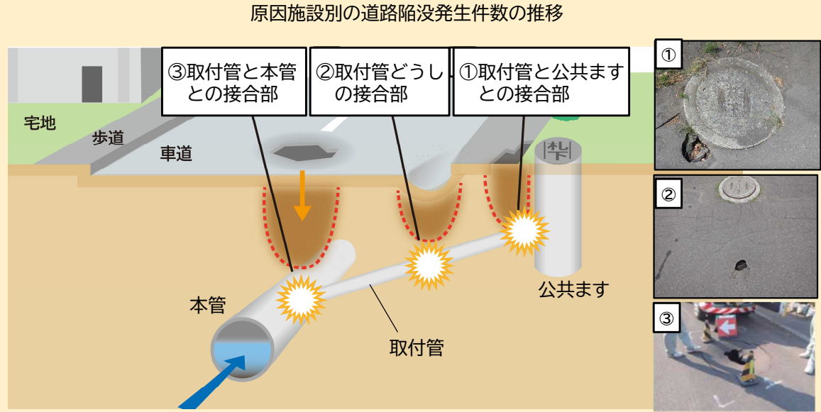
取付管による道路陥没のイメージ
