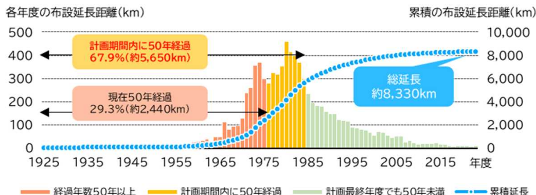
本管の年度別整備状況
