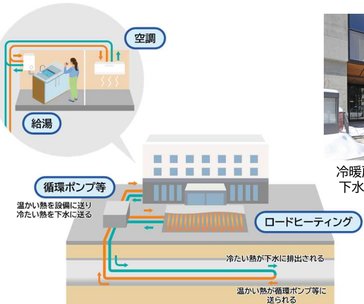
下水熱の有効利用
