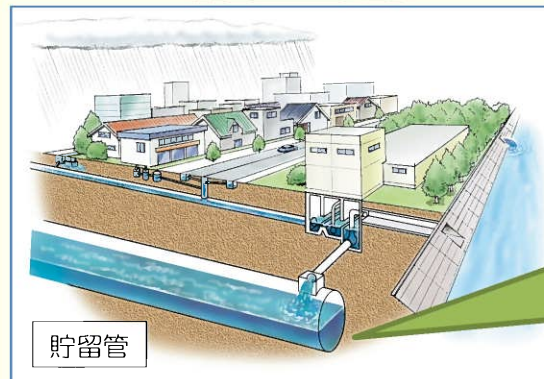
改善後(貯留管設置後)
