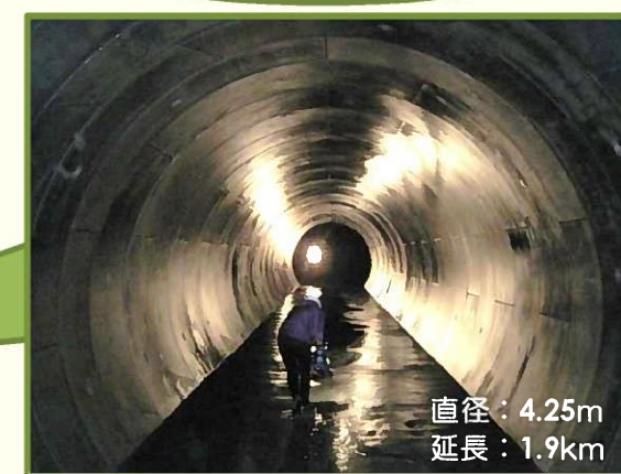
貯留管内の様子
