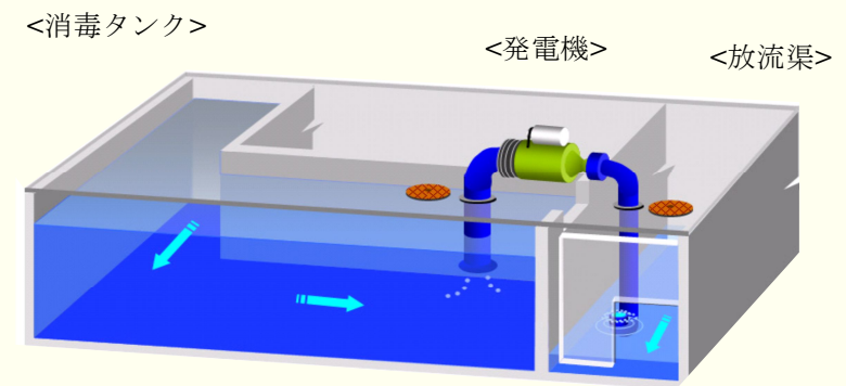
小水力発電イメージ図（サイフォン方式）
