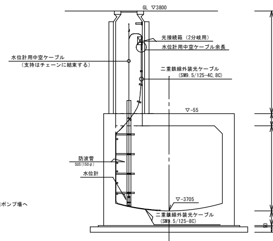
B-B断面図
