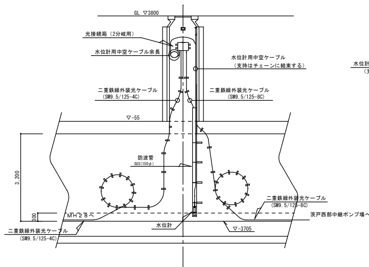
A-A断面図
