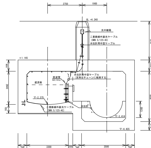
A-A断面図
