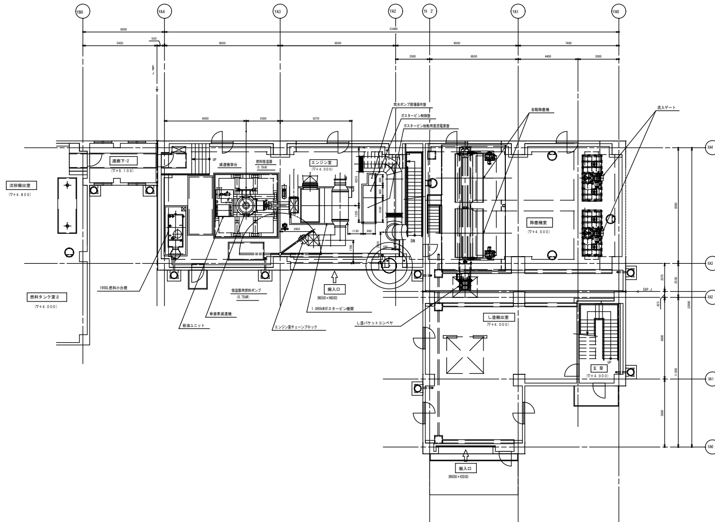
茨戸西部中継ポンプ場 雨水ポンプ施設ポンプ棟平面図（1階）
