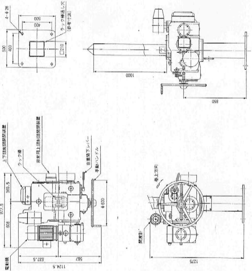
開閉装置外形寸法図（参考）
