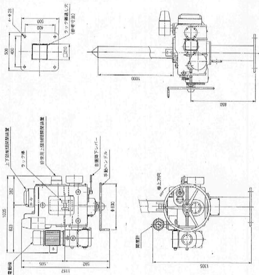
開閉装置外形寸法図（参考）
