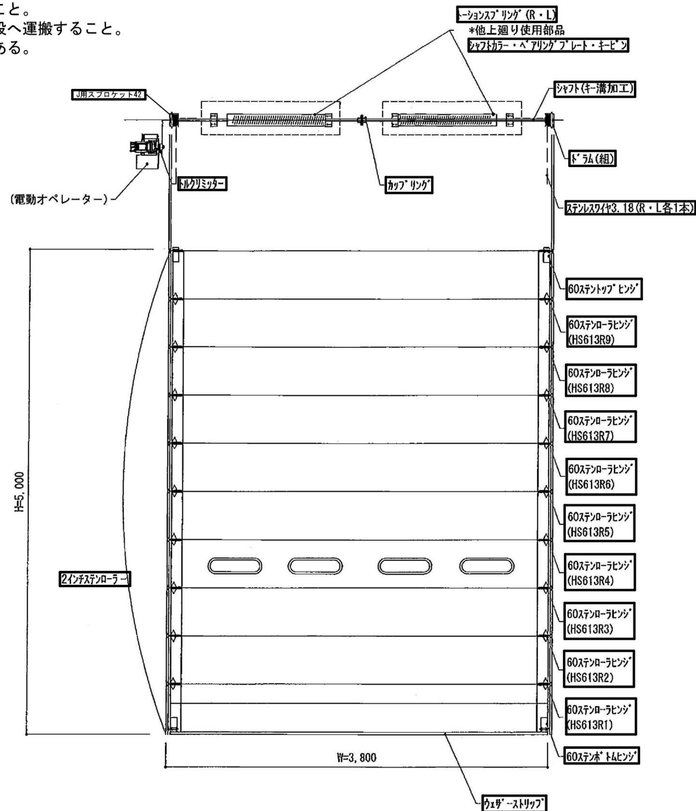
オーバースライダー詳細図 (S=Free)
