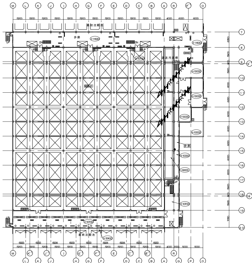
歩廊 1F 平面図
