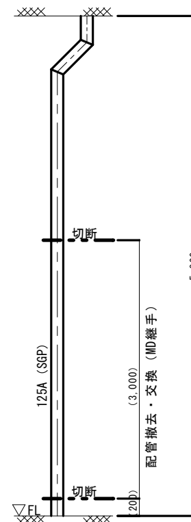
ルーフドレン配管 断面図
