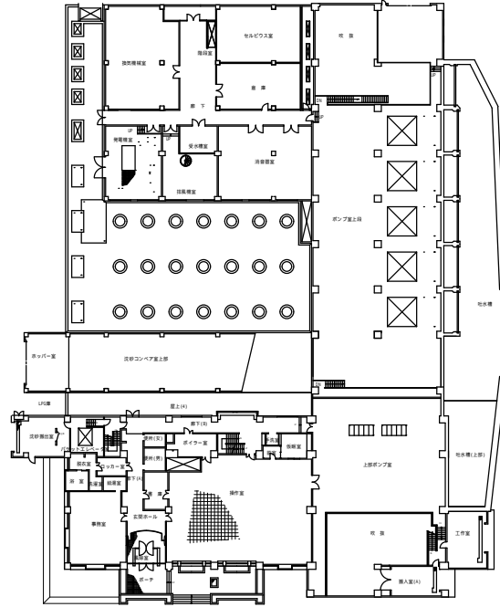
1階平面図
