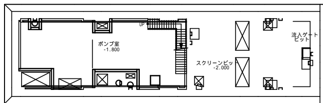
地下1階平面図
